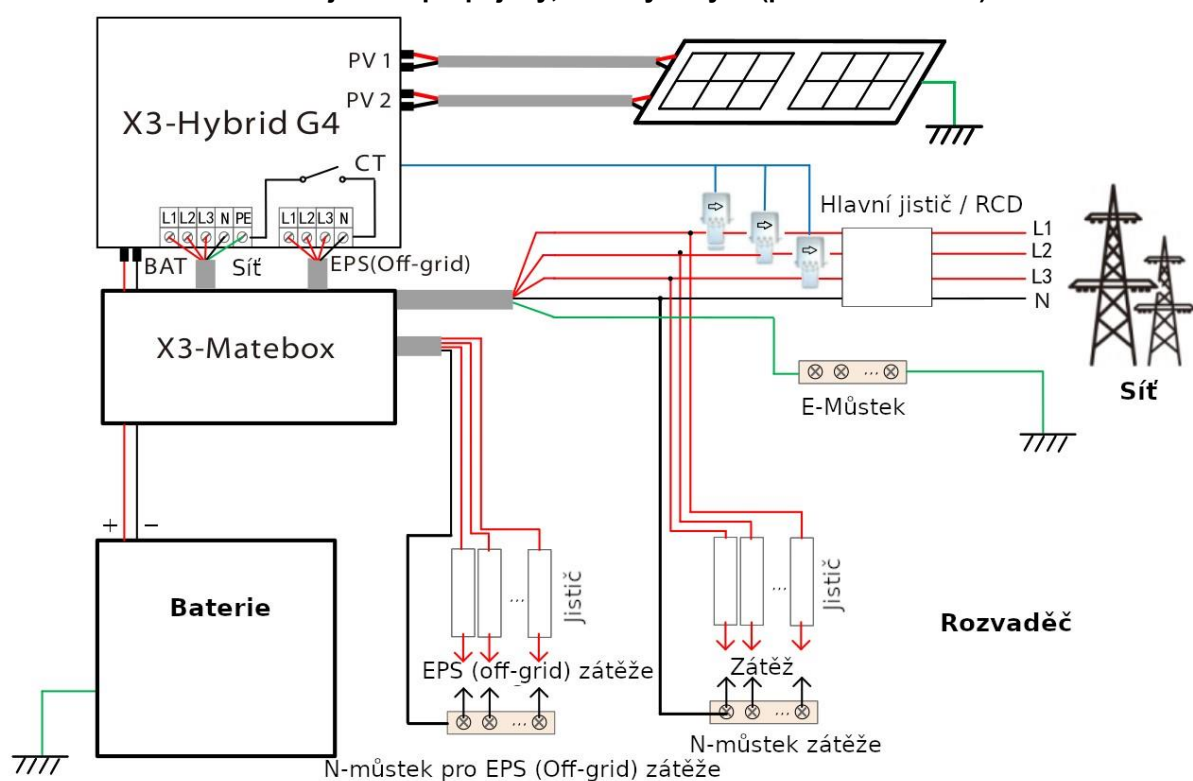
Schéma C: vodiče N a PE jsou propojeny, modely řady D (použitelné v Austrálii):
